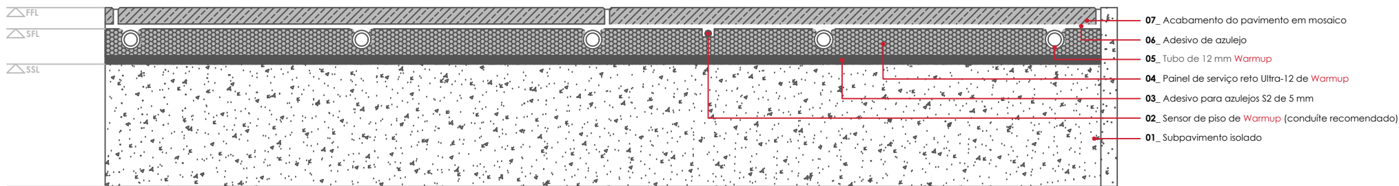
WARMUP SISTEMA ULTRA12. Acabamento do pavimento em mosaico
