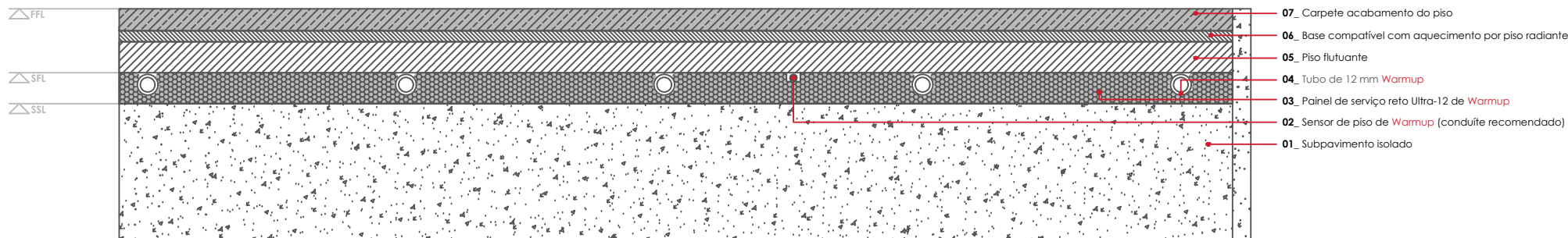
WARMUP SISTEMA ULTRA12. Carpete acabamento do piso
