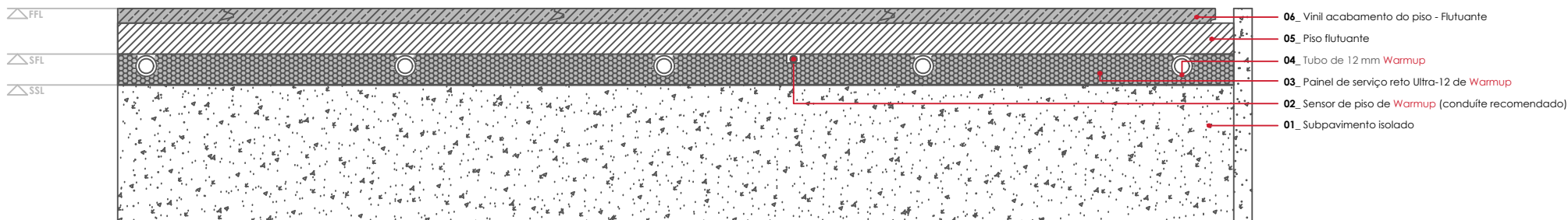
WARMUP SISTEMA ULTRA12. Vinil acabamento do piso - Flutuante
