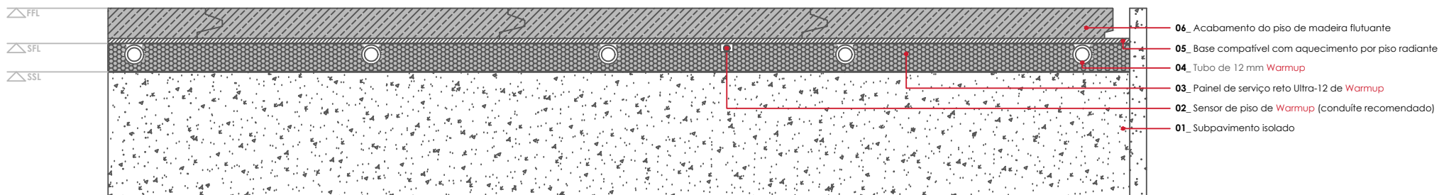
WARMUP SISTEMA ULTRA12. Acabamento do piso de madeira flutuante
