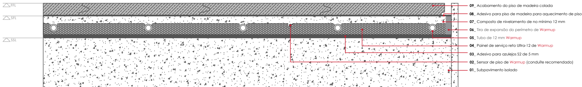
WARMUP SISTEMA ULTRA12. Acabamento do piso de madeira colada
